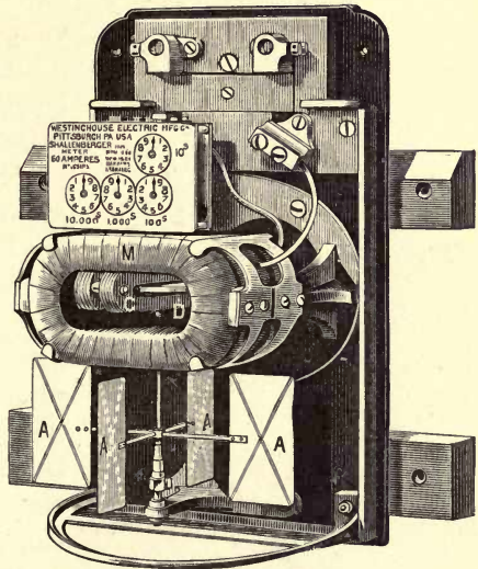
Fig. 308.—Interior of Schallenberger Meter
